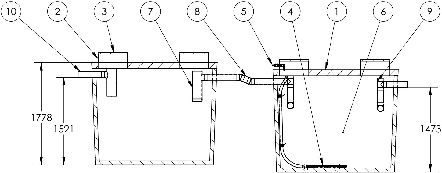
SECTION VIEW A-A BTT-1325-RO
